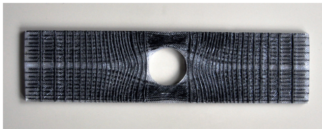
Рис. 2. Пластина с управляемой укладкой волокон
