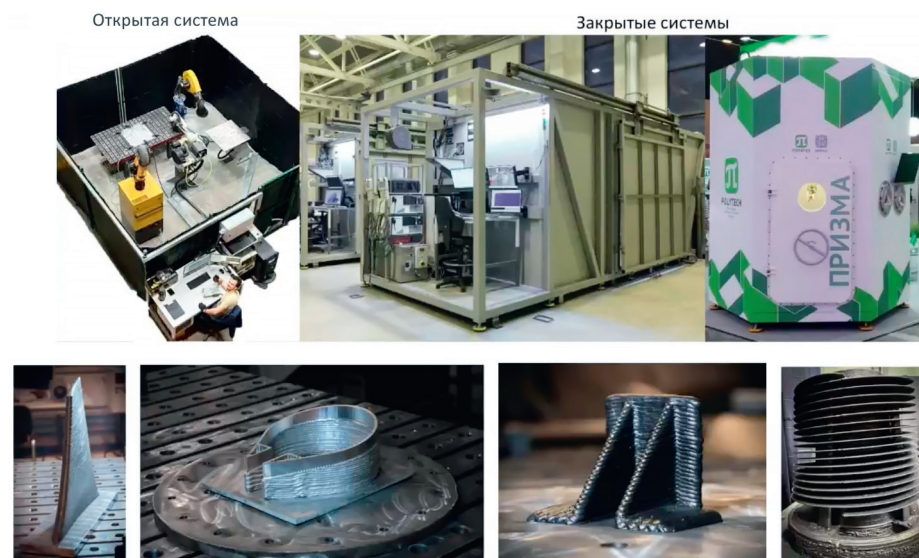
Рис. 7. Примеры разработанных систем и изделий. Фото: СПбПУ
