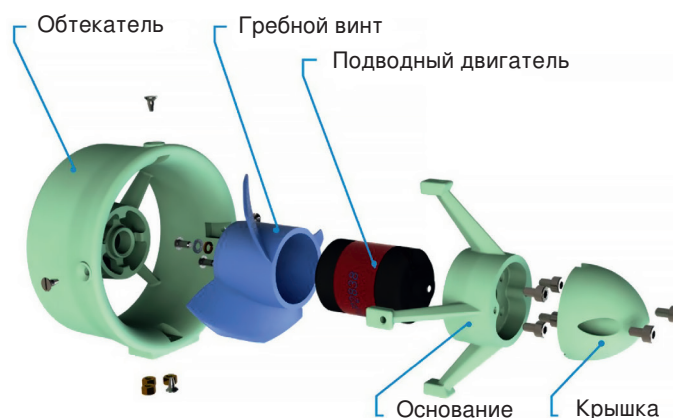
Рис. 5. Общий вид конструкции движителя
