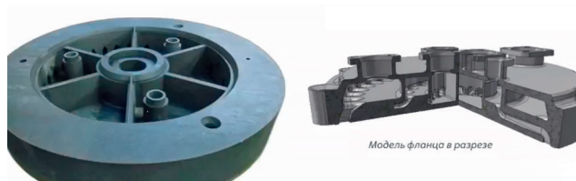
Рис. 6. Фланец электрохимического генератора/электризера, выполненный по технологии СЛМ. С помощью 3D-печати удалось в 4 раза снизить себестоимость изделия, в 3 раза сократились сроки изготовления, коэффициент использования материалов увеличен на 90%, значительно упрощена конструкция. Фото: «Росатом Аддитивные Технологии»
