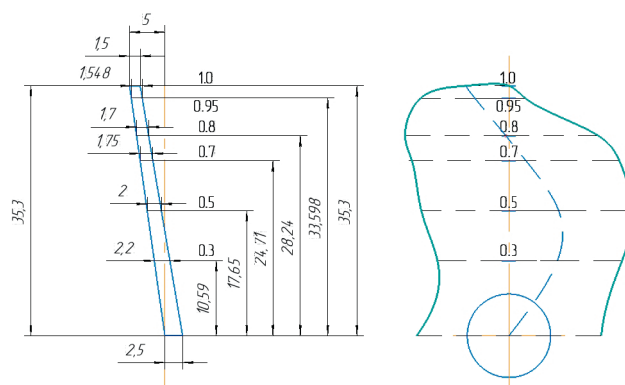
Рис. 4. Пример построения профиля лопастей
