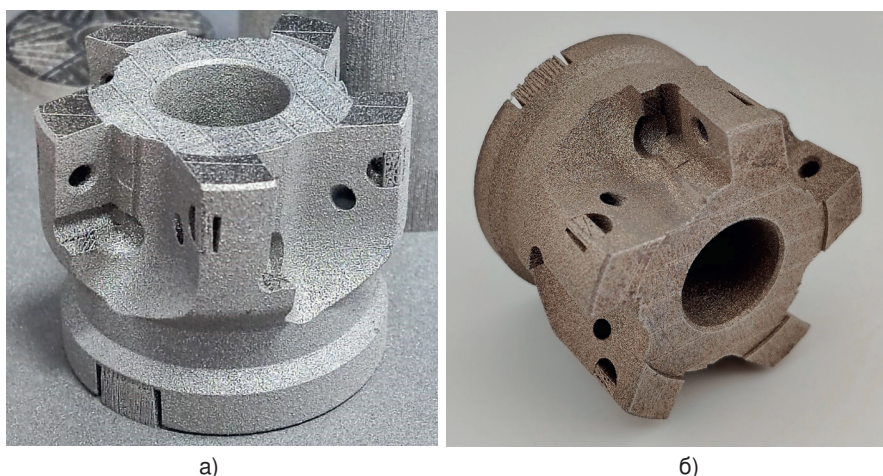
Рис. 14. Внешний вид корпуса фрезы после аддитивного построения: а — на подложке as built; б — перед удалением поддержек
