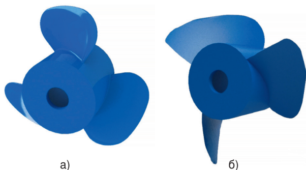
Рис. 2. Общий вида (а) непрофилированного гребного винта и (б) профилированного гребного винта с углом поворота (наклона) 40 градусов
