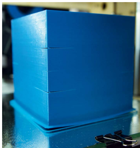
Рис. 3. Куб 10×10×10 см с заполнением 5%, напечатанный из ABS и AEROTEX
