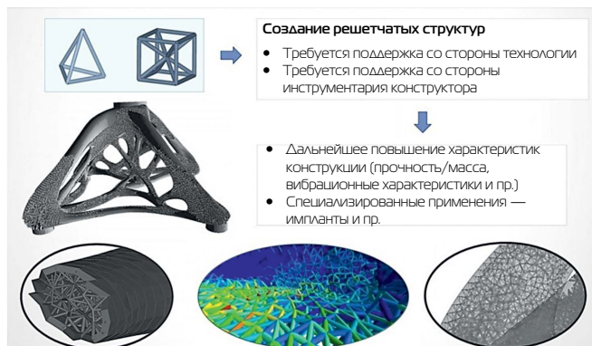
Рис. 2. Создание решетчатых структур
