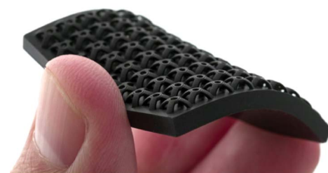
Образец сложной текстуры с подрезками
