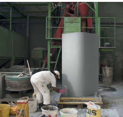
Рис. 14. Пример сетчатой структуры, заполненной бетоном с ручной финишной отделкой
